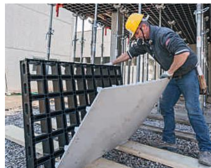
2. Entfernen der beschädigten Schalhaut
