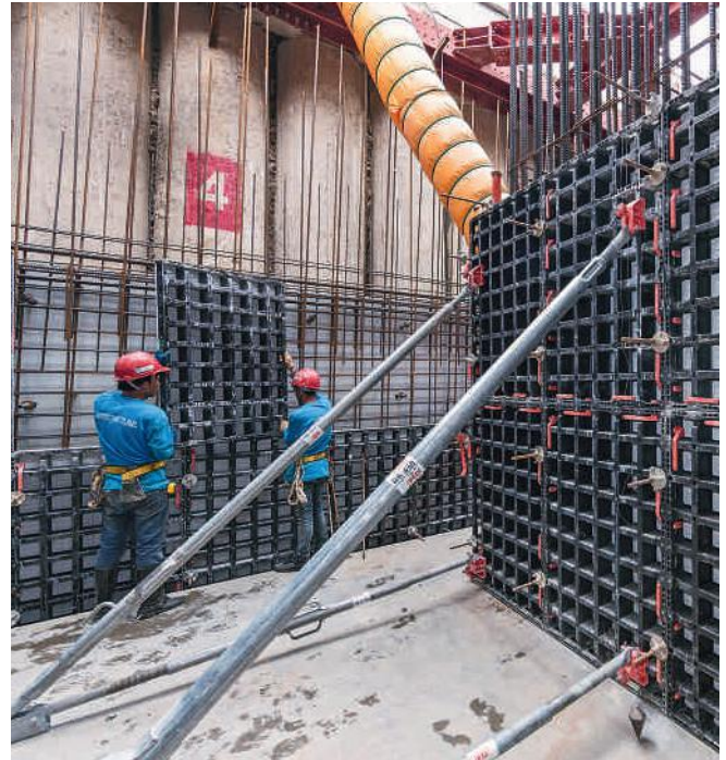
Geringes Gewicht, kleinformartige Schalungselemente – diese Vorteile spielt DUO bei diesen Tiefgeschosswänden voll aus
